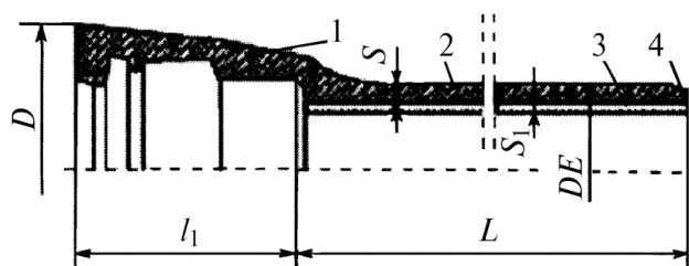
1 – раструб; 2 – тело; 3 – ЦПП; 4 – фаска
