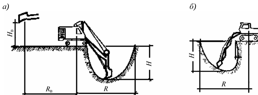
а) – система управления канатная; б) – система управления гидравлическая
