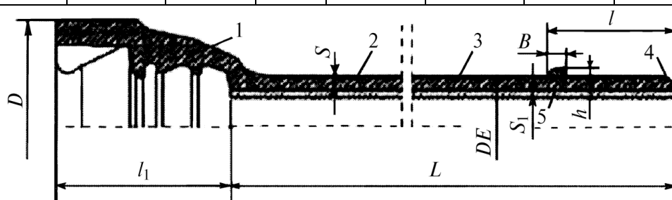
1 – раструб; 2 – тело; 3 – ЦПП; 4 – фланец; 5 – наплавленный выступ
