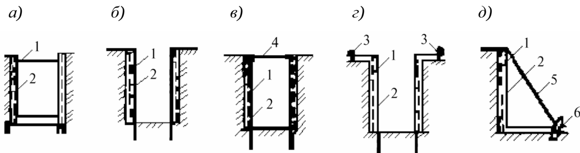
а) – распорное; б) – консольное; в) – консольно-распорное; г) – консольно-анкерное; д) – подкосное; 1 – щиты; 2 – стойки (сваи); 3 – анкера; 4 – распорки; 5 – подкосы; 6 – упоры
