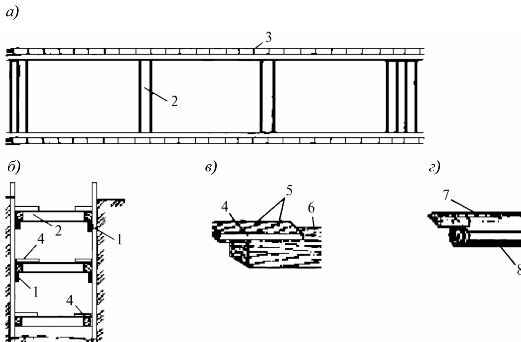
а) – вид сверху; б) – вид вдоль траншеи; в), г) – узлы сопряжения элементов креплений; 1 – бобышка; 2 – распорка; 3 – доски толщиной 50 мм; 4 – накладка из доски; 5 – гвозди; 6 – брус 100 мм; 7 – накладка из горбыля; 8 – бревно
