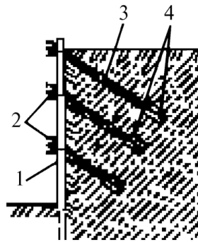
1 – шпунтовая стенка; 2 – балки; 3 – тяги; 4 – анкеры
